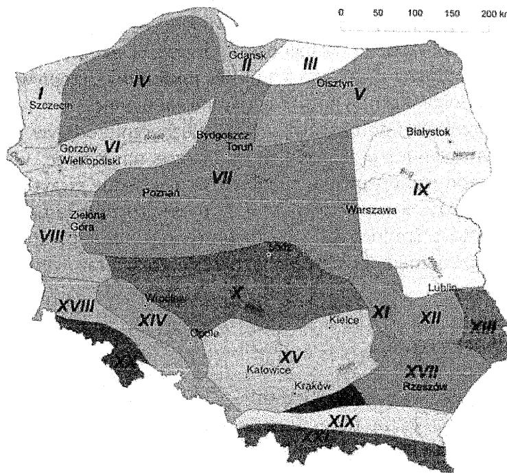
Rysunek: Dzielnice rolniczo-klimatyczne Polski wg R. Gumińskiego
